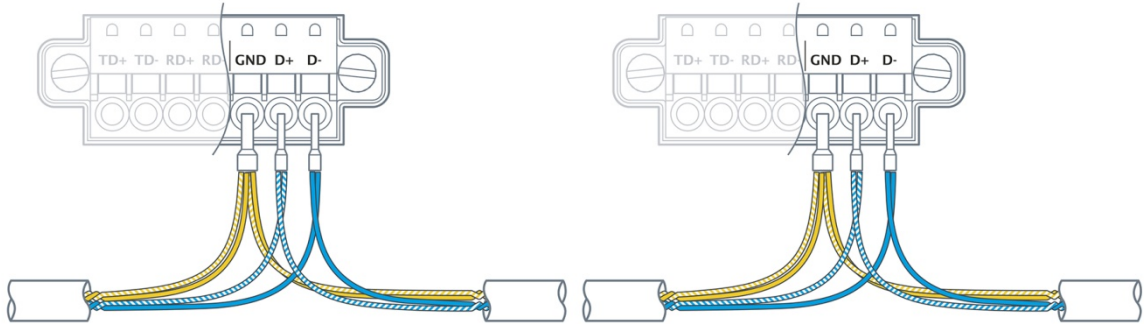
Рис. 31 - Организация сети RS-485
