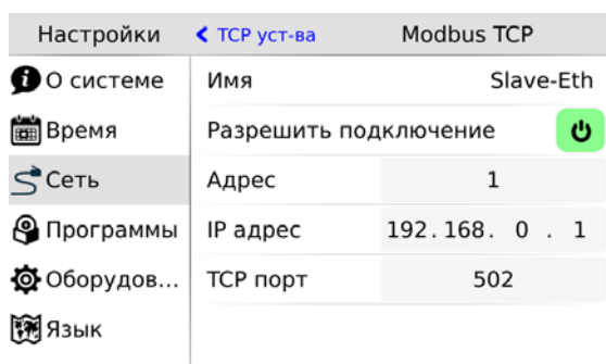
Рис. 60 – Настройка Modbus TCP slave
