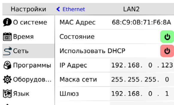
Рис. 54 - Редактор настроек интерфейсов Ethernet
